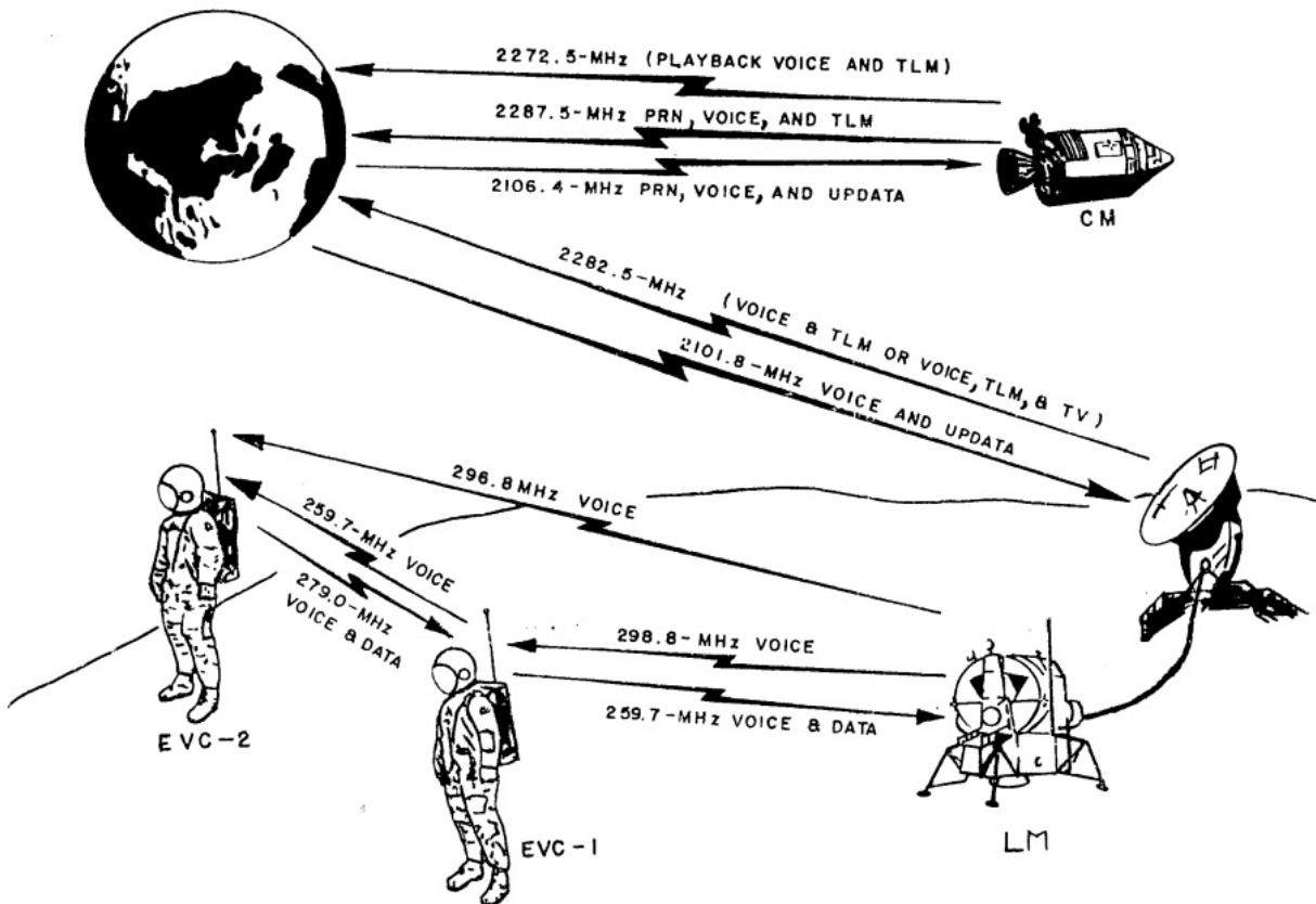
Abbildung 12: Übersicht der Funkverbindungen zwischen Apollo 11 und der Erde (Bild: NASA, Corliss (1974)).
